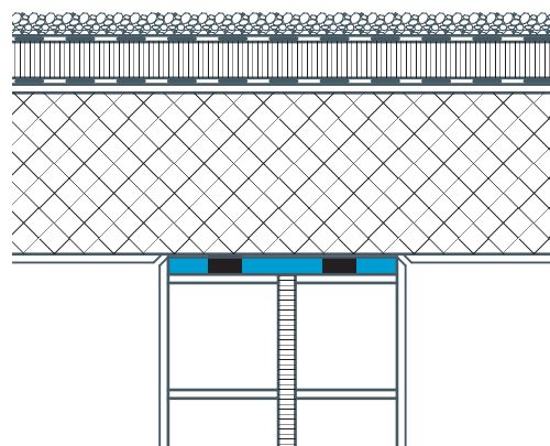
→ Muro con intercapedine con soletta continua
