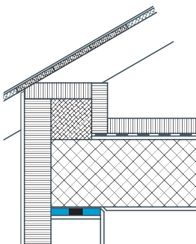
→ Isolamento facciata / tetto spiovente
