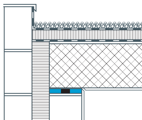
→ Muratura doppia
