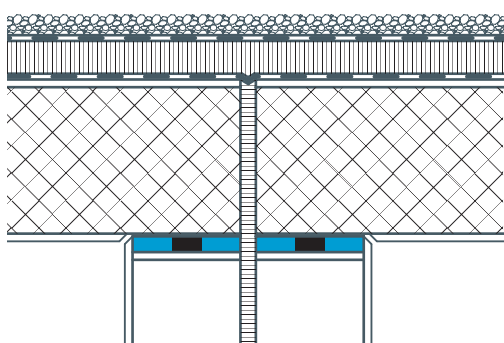
→ Giunto di dilatazione dell'edificio
