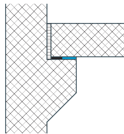
→ Appoggio per mensola
