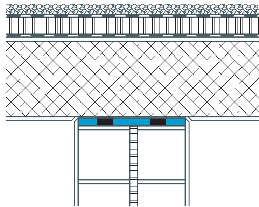
→ 2-schalige Wand mit durchlaufender Decke
