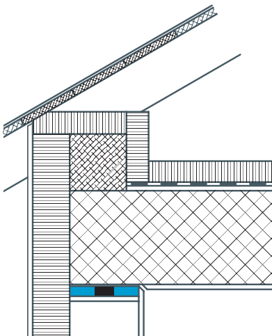
→ Fassadenisolation / Steildach
