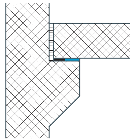
→ Konsolen-Auflage
