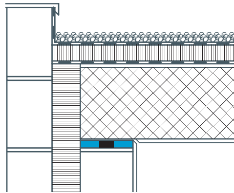
→ Zweischalen-Mauerwerk
