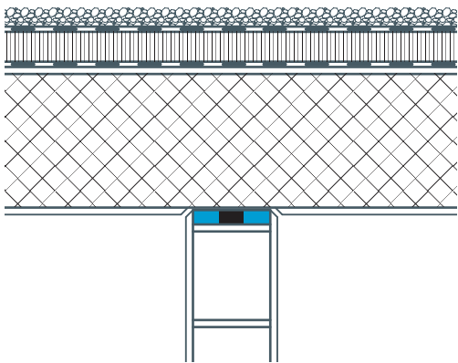
→ Tragende Zwischenwand
