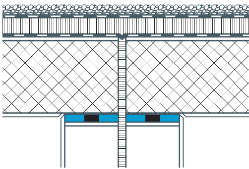
→ Gebäudedilatation
